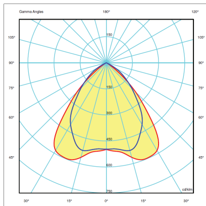
I LUM 85x85: Bisimetrična raspodjela svjetla prema dolje 85x85°.
