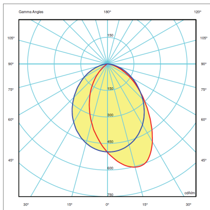
I LUM 60x90: Asimetrična raspodjela svjetla prema dolje 60x90°
