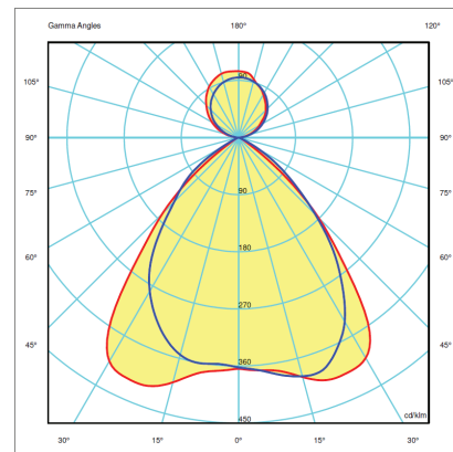
I LUM 85x85 + PREMA GORE: Bisimetrična raspodjela svjetla prema dolje 85x85° + simetrična raspodjela svjetla prema gore 110°.
